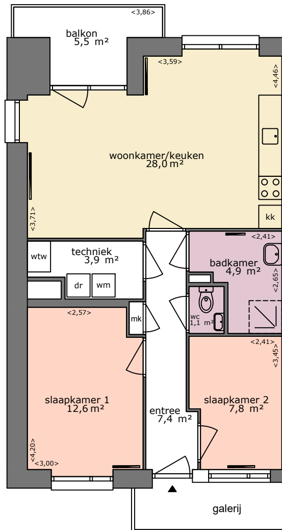
3e verdieping
