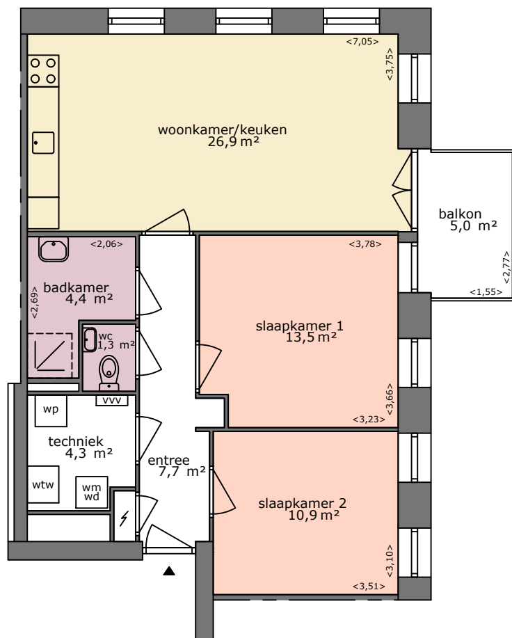
Appartement 4e verdieping
