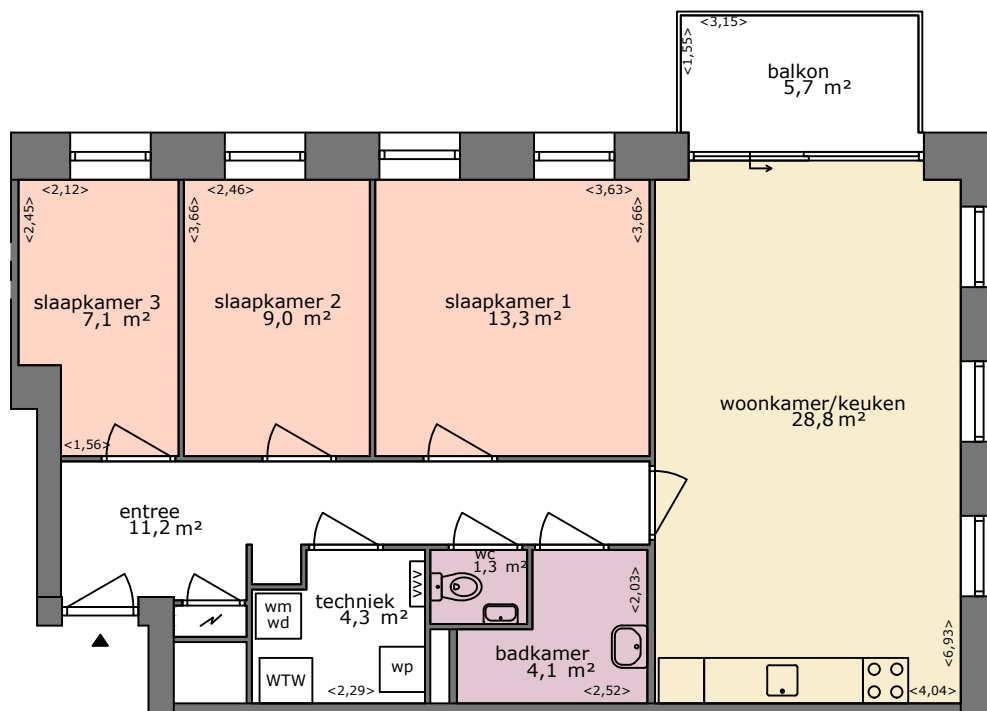
Appartement 2e verdieping
