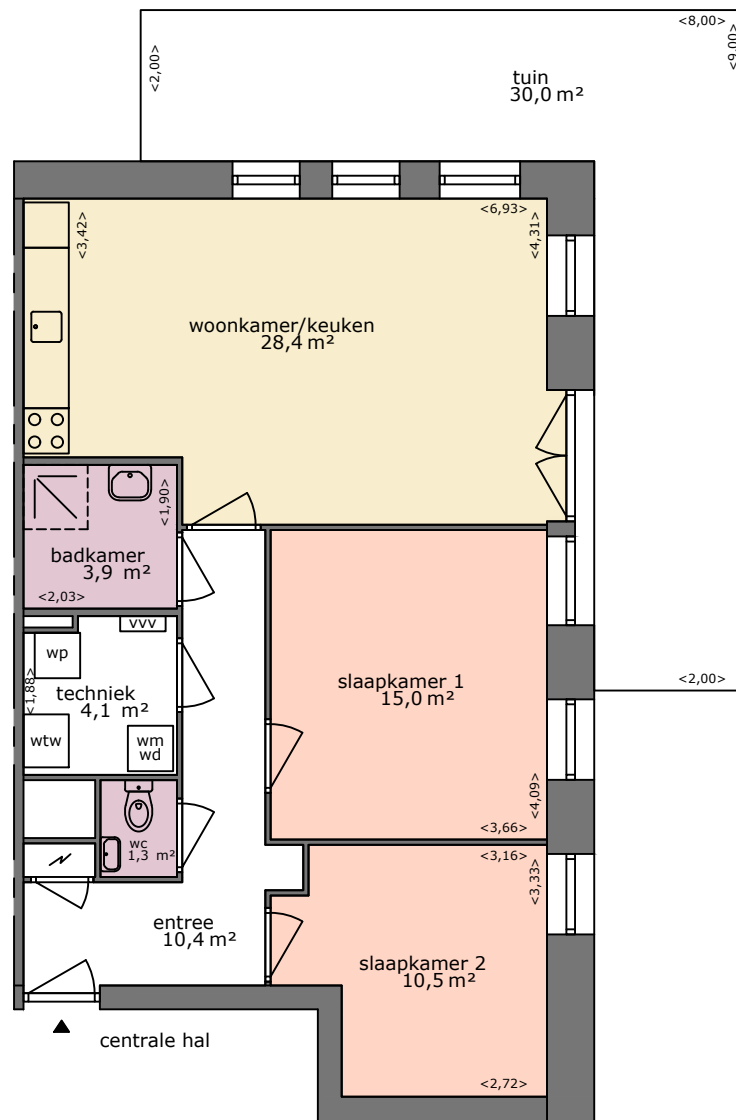
Appartement begane grond
